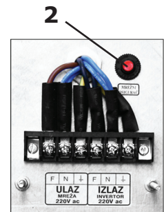
Izgled priključne kutije sa rasporedom klema
